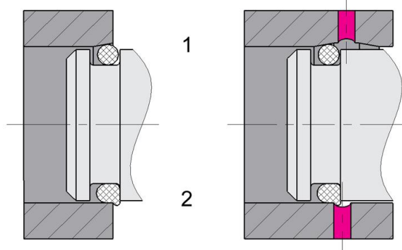
Fig. 6: Instalación a través de chaflán de entrada y orificio transversal
