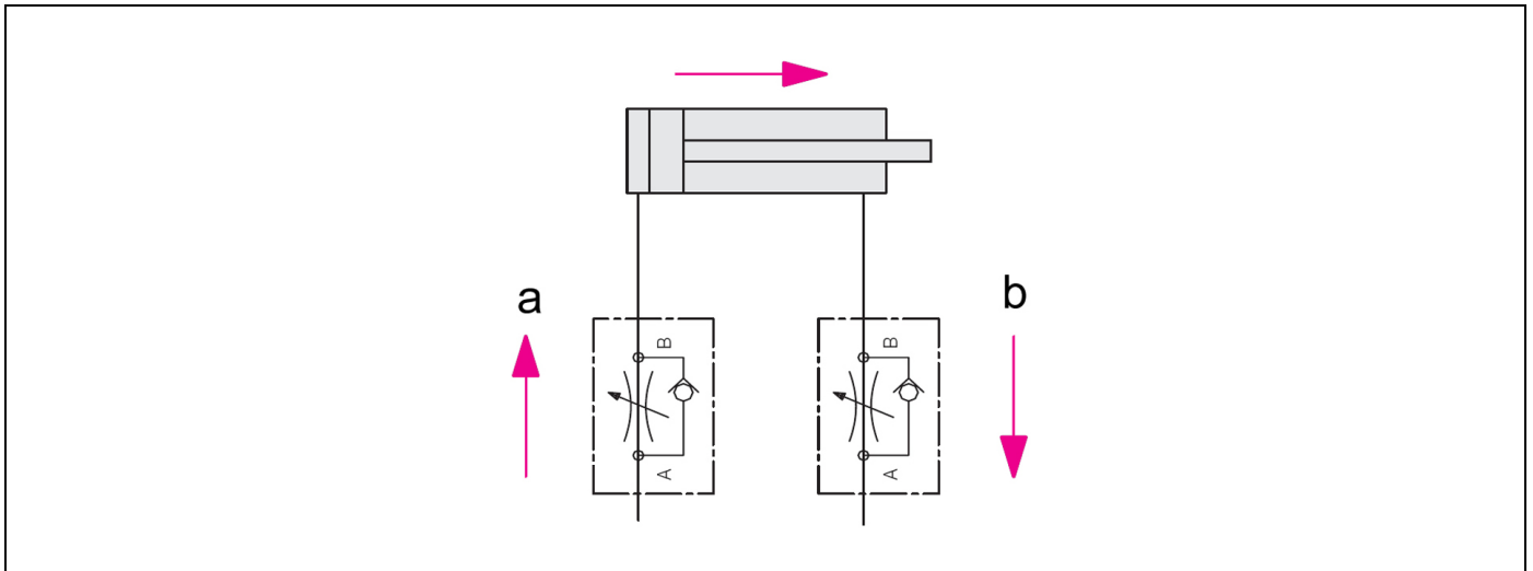
Fig. 4: Esquema hidráulico con válvula estranguladora con válvula antirretorno
