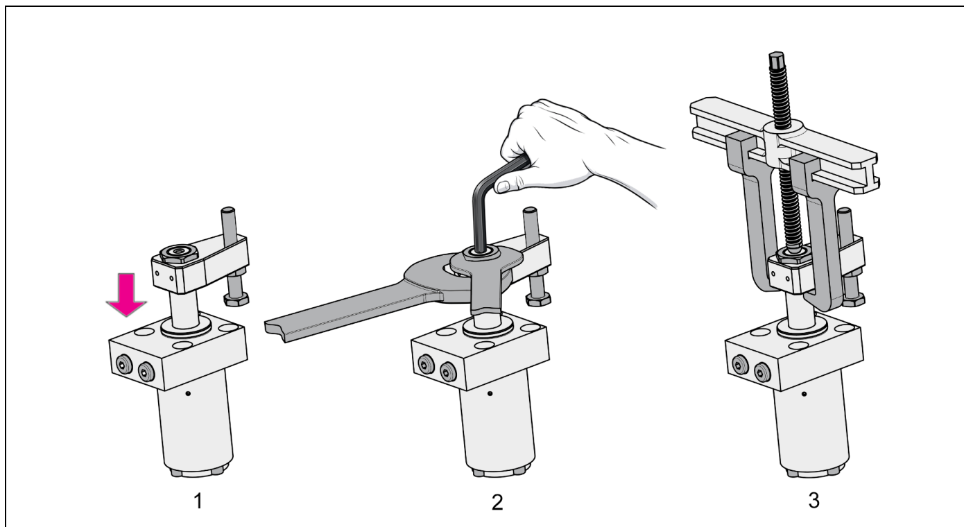
Fig. 7: Montaje / desmontaje - ejemplo
