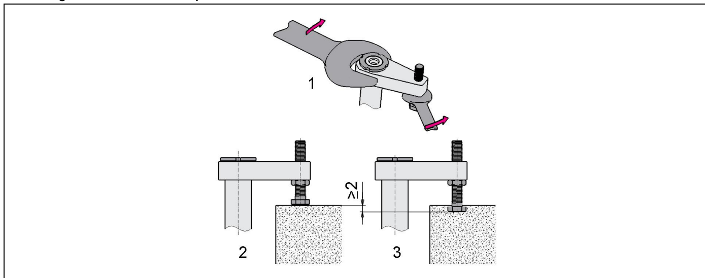
Fig. 8: Regulación de la brida de sujeción - ejemplo
