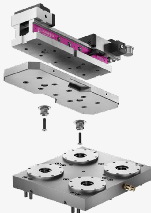
Fixation avec pions de serrage avec plaque d'adaptation dans le système de serrage point zéro
