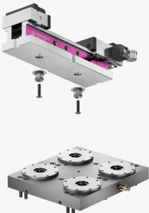
Fixation avec pions de serrage directement dans le système de serrage point zéro
