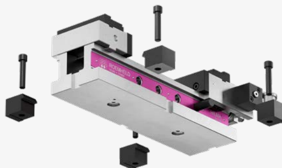
Fixation avec griffe de serrage (Recommandation : distance des griffes de serrage < 200 mm)
