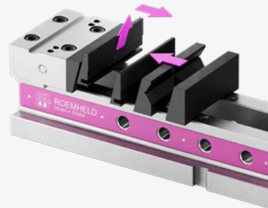
QIS-Wechselbacke bis Nutende hochschieben und abkippen
