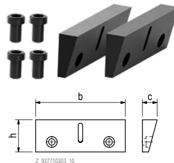
QIS-Wechselbacke bis Nutende hochschieben und abkippen
