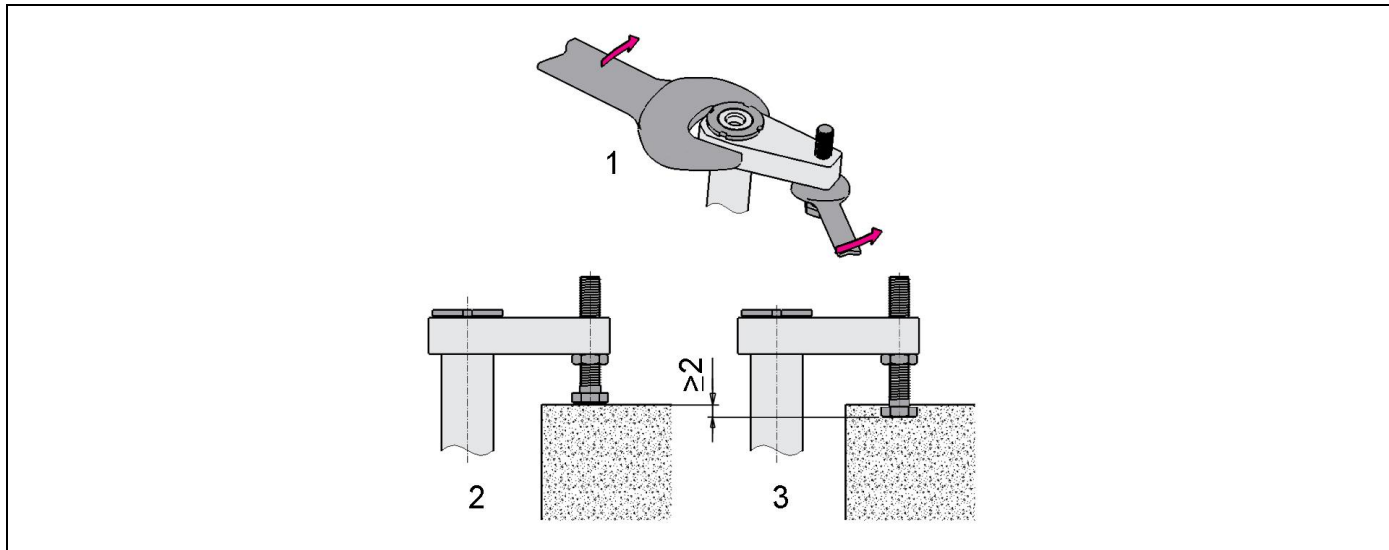
Fig. 8: Exemple du réglage de la vis de pression
