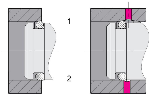
Fig. 6: Installation par chanfrein d'entrée et alésage transversal
