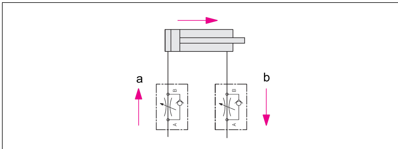
Fig. 4: Schéma hydraulique avec étrangleurs
