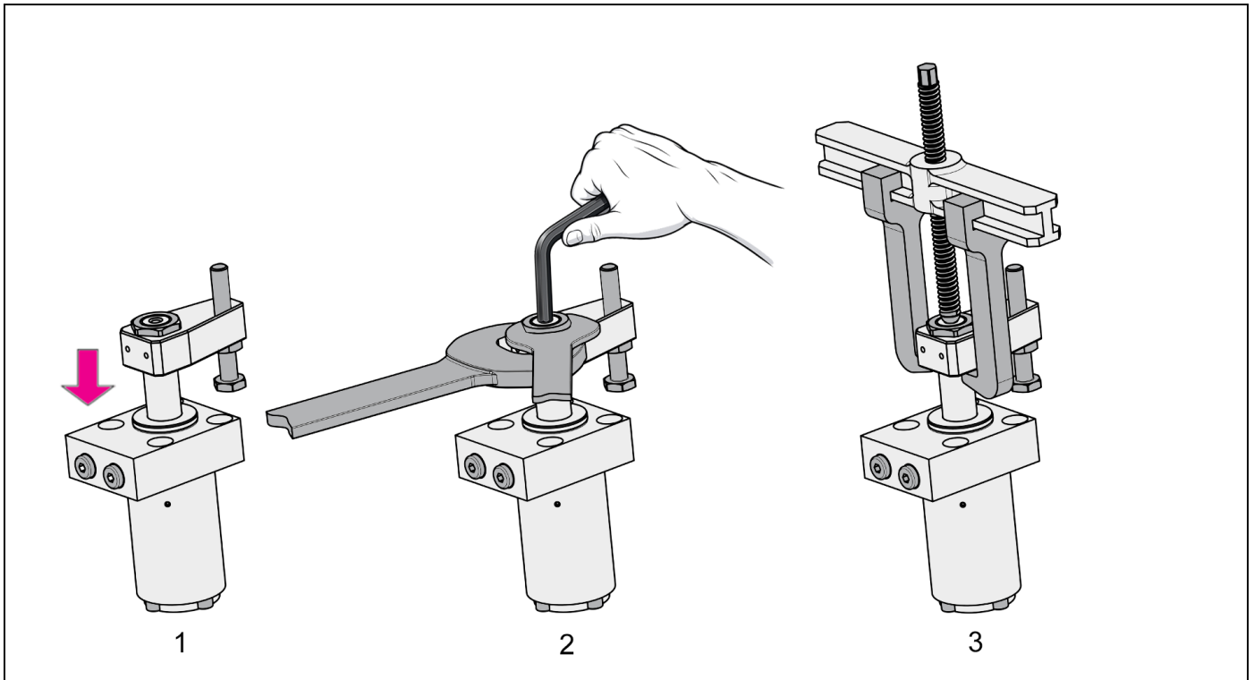
Fig. 7: Montage / démontage - exemple
