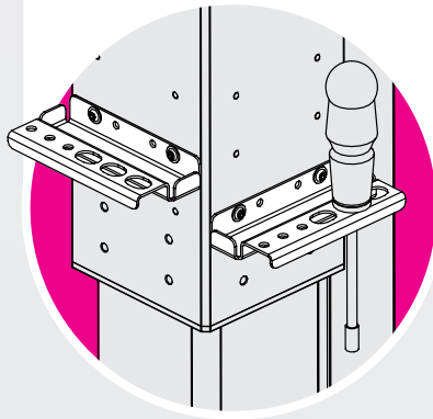
Werkzeughalter
