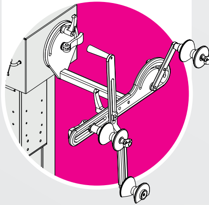
3-Punkt-Aufnahme
