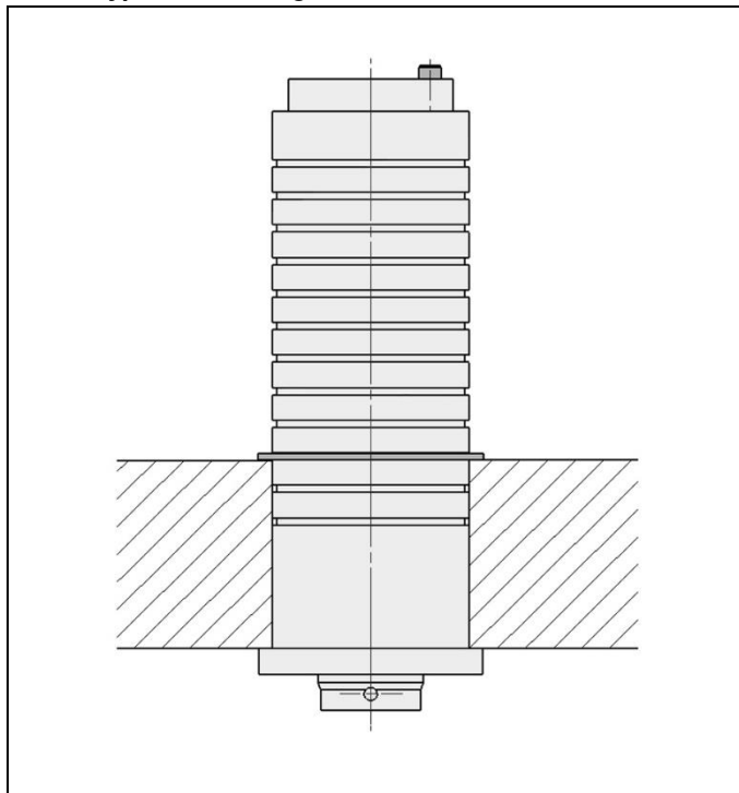
Fig. 2 : Possibilité de fixation
